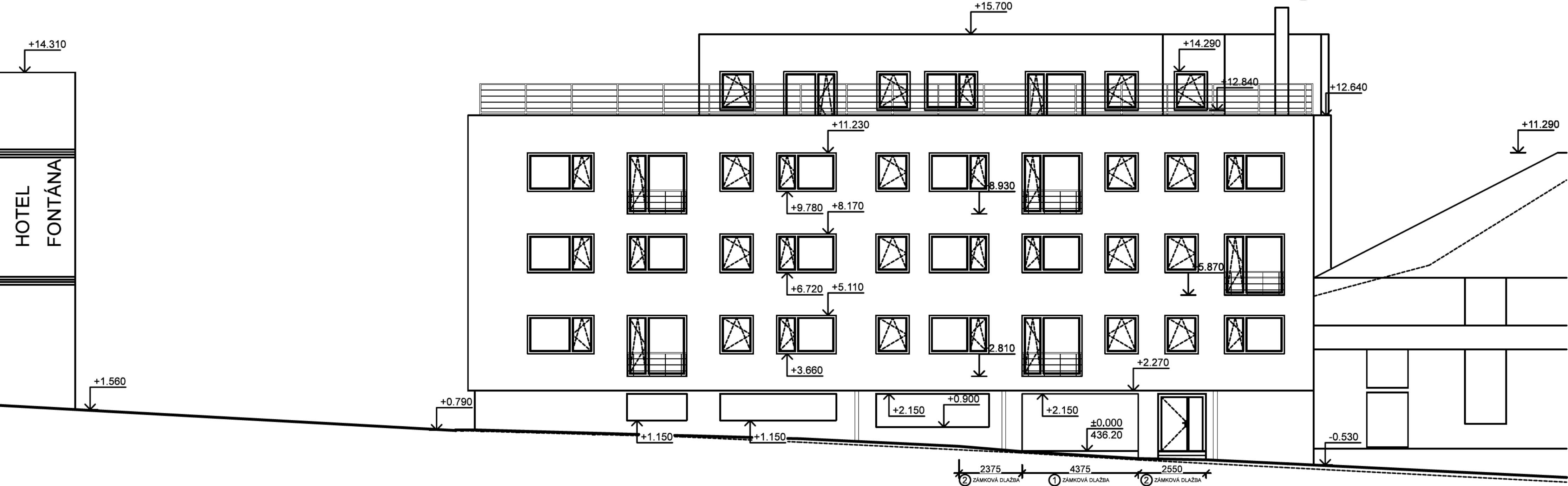
POHLED JIŽNÍ
