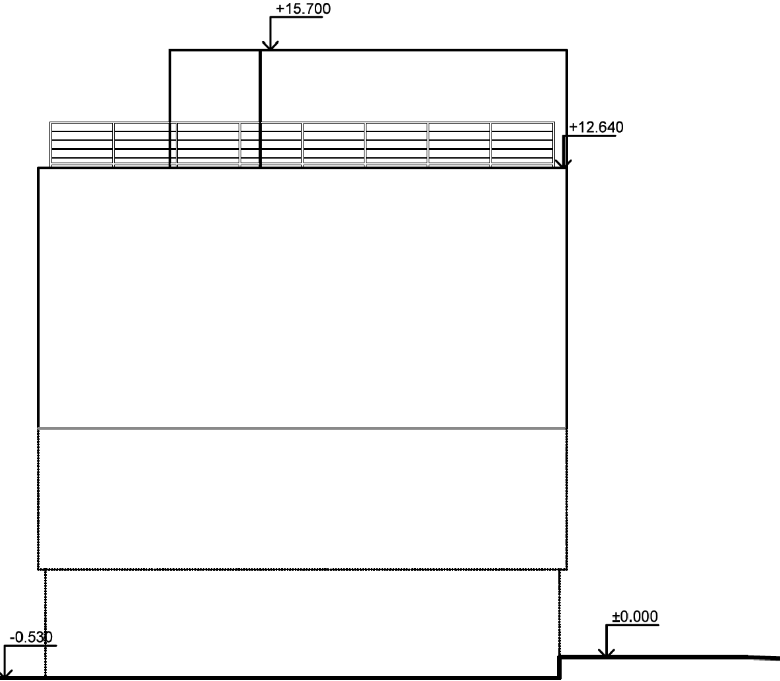
POHLED VÝCHODNÍ
