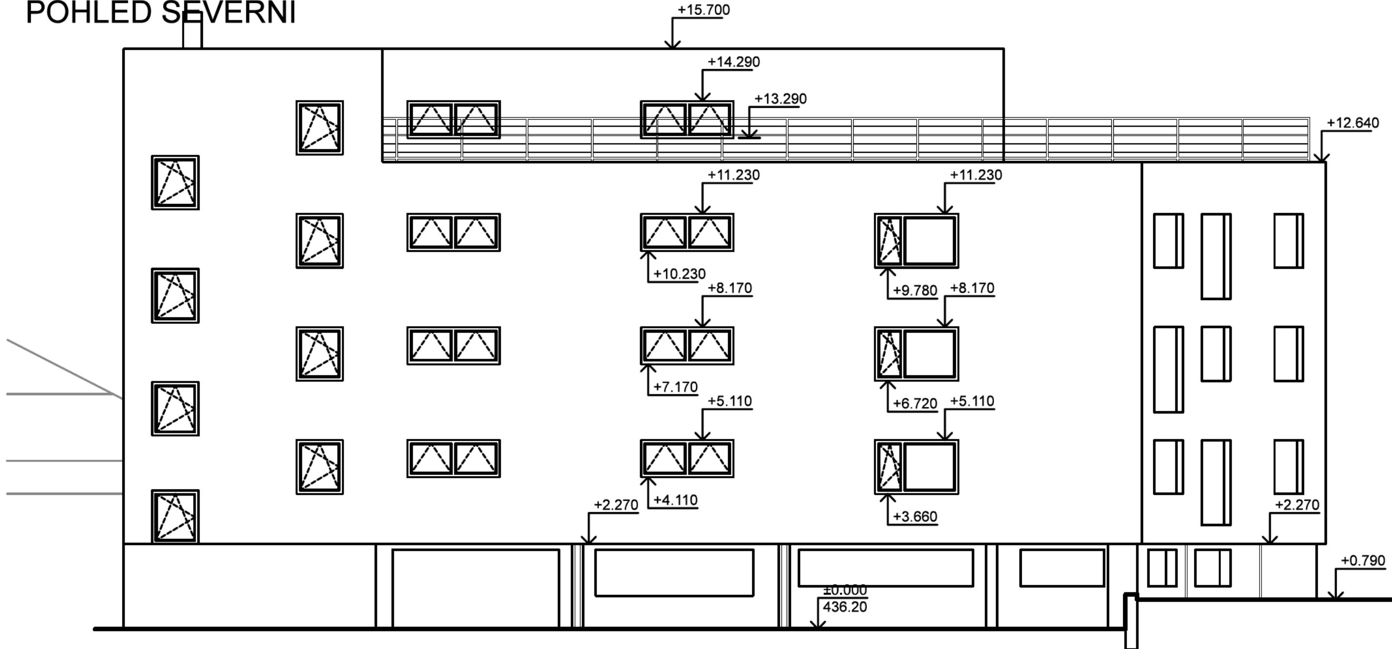
POHLED SEVERNÍ
